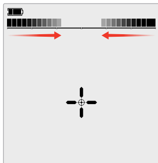
Sinyal target lemah/di luar pusat: Lebih sedikit segmen diskriminasi yang Aktif. Target terletak lebih dekat ke bagian luar coil.
